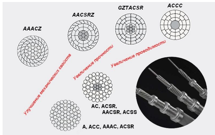
Рис.1 Эволюция проводов для ВЛ.
